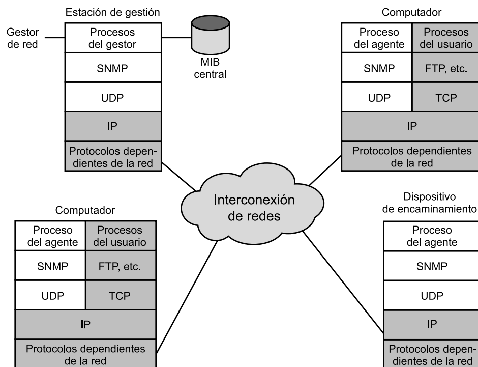
Figura 22.7. Configuración SNMPv1.
