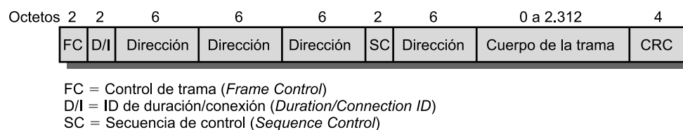
Figura 17.8. Formato de la trama MAC en IEEE 802.11.
