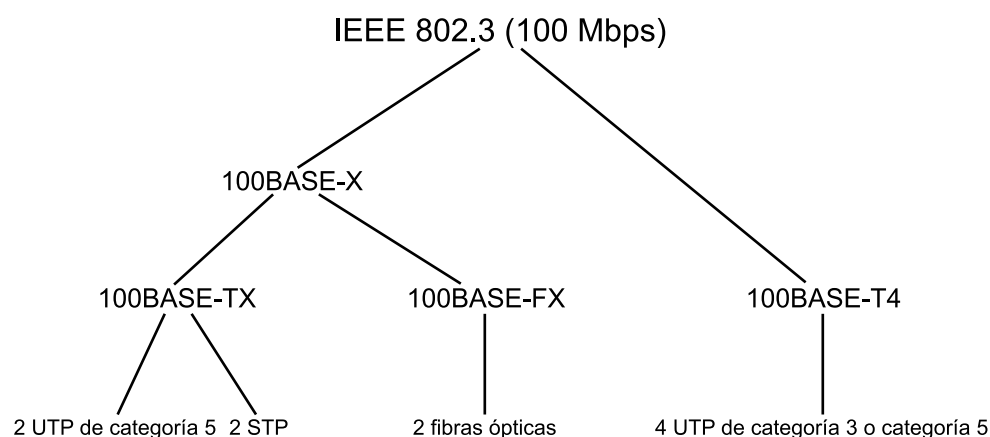
Figura 16.4. Opciones 100BASE-T en IEEE 802.3.
