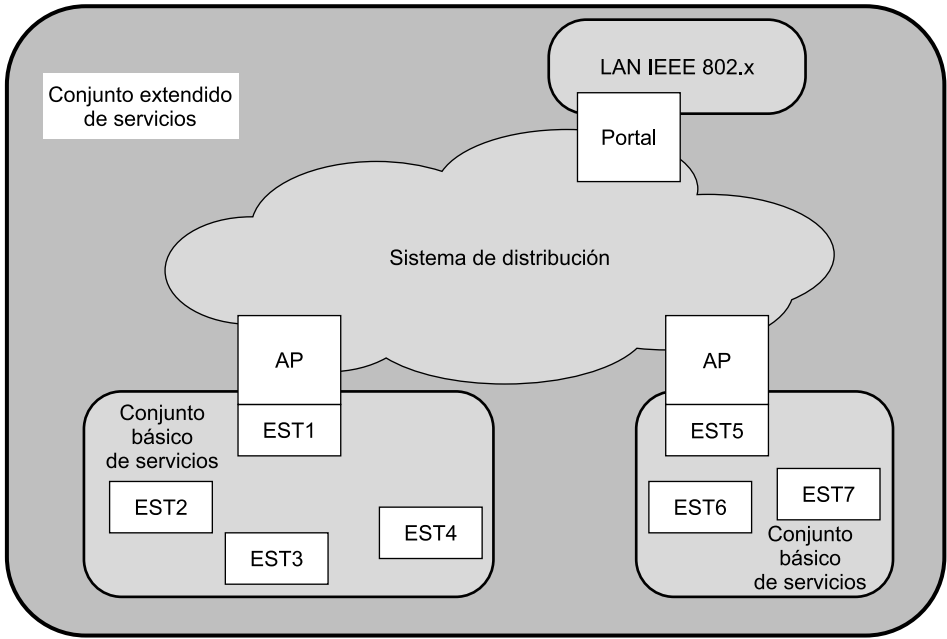
Figura 17.4. Arquitectura IEEE 802.11.
